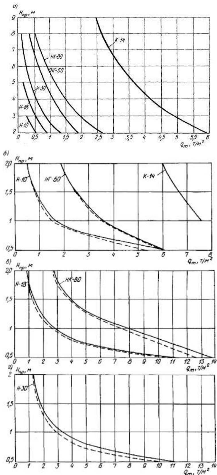
Рисунок 4.1. Зависимость нормативного давления от транспорта q_m от глубины заложения трубопровода H_{зр} , при диаметре труб 110 мм (сплошные линии), при диаметре труб 500 мм (пунктирные линии)
