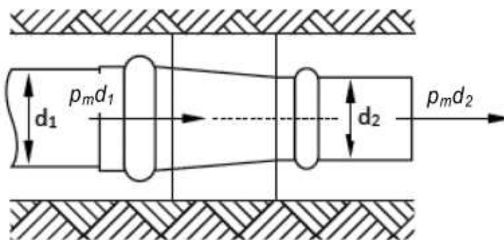
Рисунок 4.3. Опорный блок переходного патрубка
