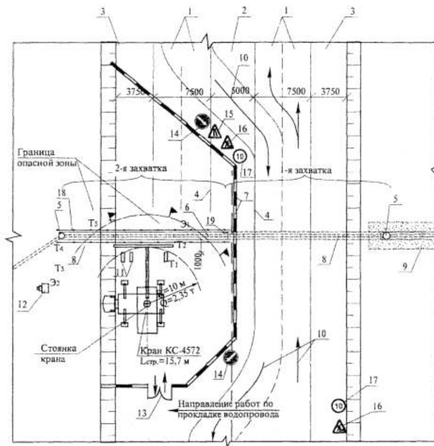
Рисунок 5.7 – Схема организации рабочего места при укладке трубопровода при переходе его через проезжую часть (левая сторона проезжей части автодороги) 1 – проезжая часть, полосы движения; 2 – разделительная полоса; 3 – обочина; 4 – дорожный барьер; 5 – водопроводные колодцы; 6 – проектируемый переход водопровода; 7 – дорожные тумбы; 8 – трубы водопроводные; 9 – проложенный участок водопровода; 10 – направление движения автотранспорта; 11 – лежни; 12 – сварочный агрегат; 13 – ворота; 14 – импульсная стрелка; 15 – сужение дороги (налево, направо); 16 – дорожные работы; 17 – ограничение скорости; 18 – ограждение траншеи и участка работ; 19 – лестница для спуска в траншею. Т1, Т2, Т3, Т4, Э1, Э2 – рабочие места исполнителей.
